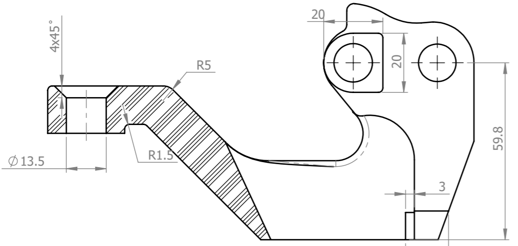
SECTION A-A SCALE 1 : 1.3
